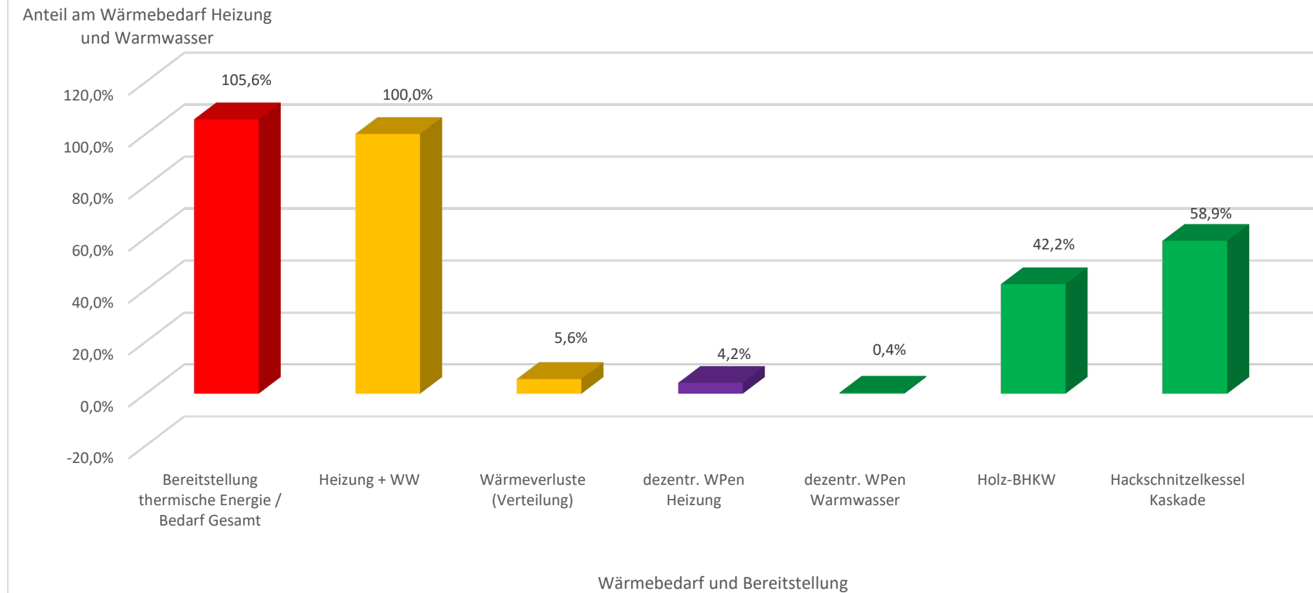
Jährliche Wärmeerzeugungsanteile prozentual zum Gesamtwärmebedarf - Variante A
