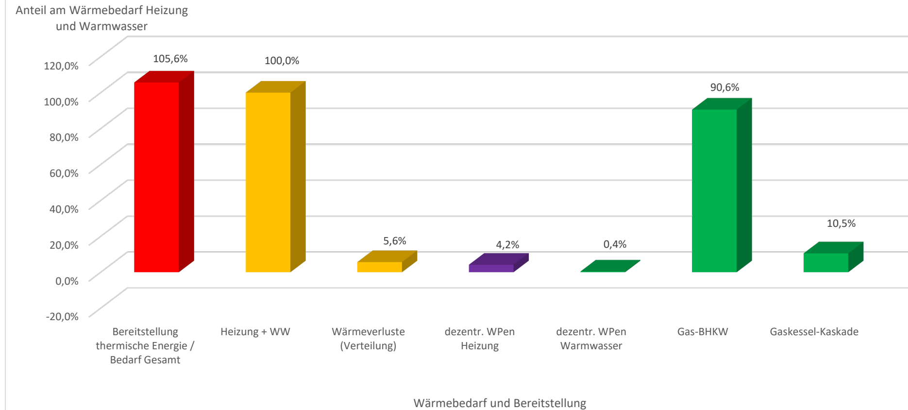
Jährliche Wärmeerzeugungsanteile prozentual zum Gesamtwärmebedarf - Variante B
